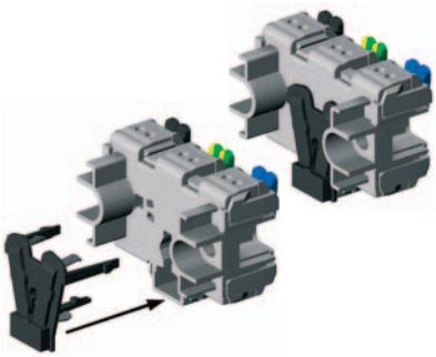
Einsetzen des Beleuchtungszusatzes.
