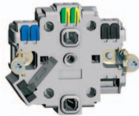
2fach-Steckdose
