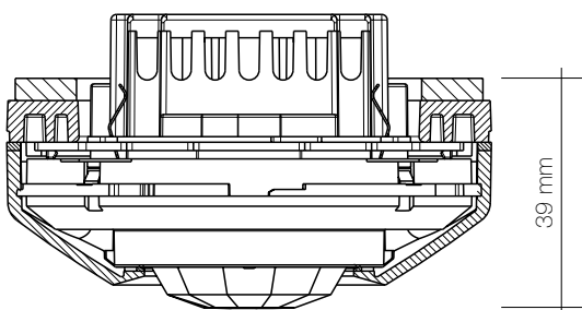
Querschnitt piriOS 360° NASS
